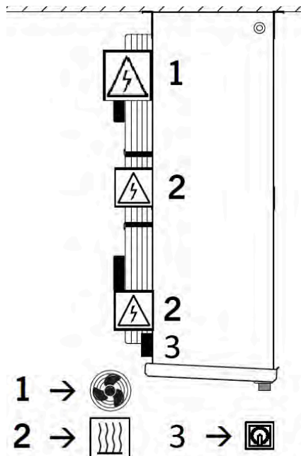
Montage Blockheizung
