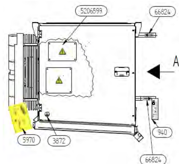
Seitenansicht links
