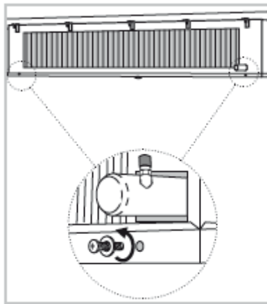
Montage der Wannenheizung
