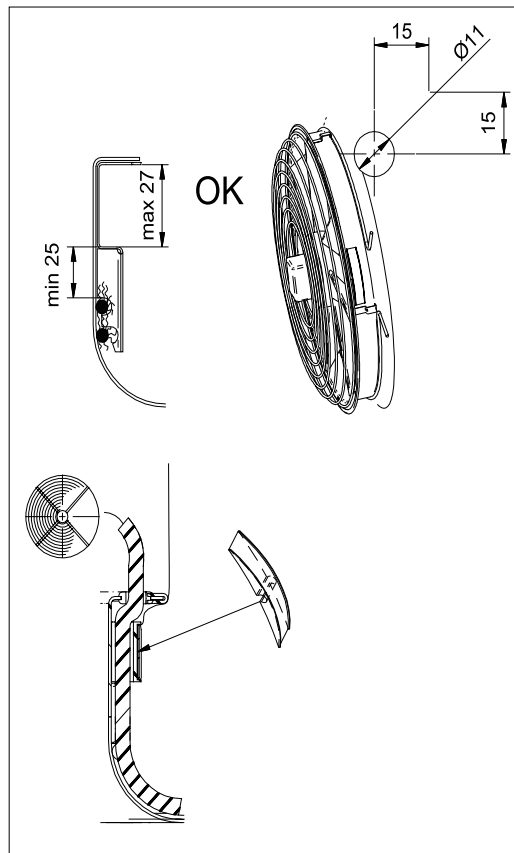
5970 - Anhänger Luftschlauchanschluss (nur bei optionalem Luftschlauchanschluss) Nur an GHN 071.2 - 080.2 mit optionalem Luftschlauchanschluss
