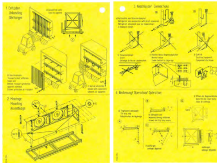
5964 - Anhänger für Entladung
