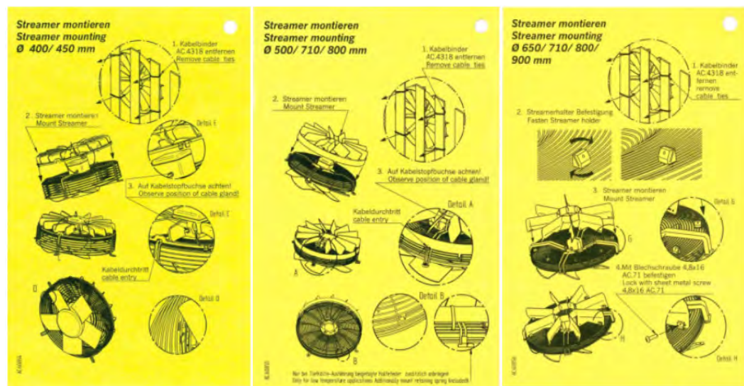
60854, 60855 und 60856 - Anhänger für Streamer Montage
