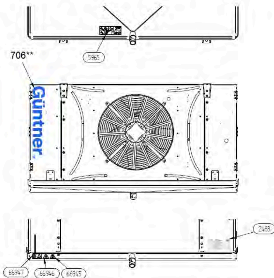
Frontansicht und Wanne Lamellenseite
