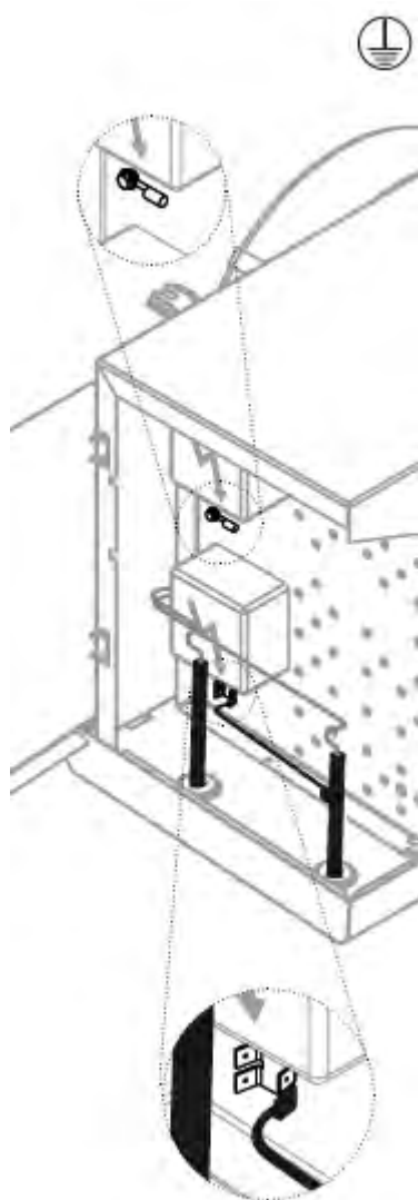
Erdung
